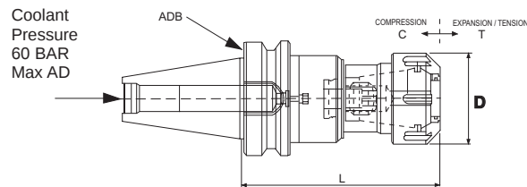
Style B — V-Flange &amp; BT
